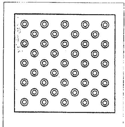
点字ブロック運輸点 300mm × 300mm
