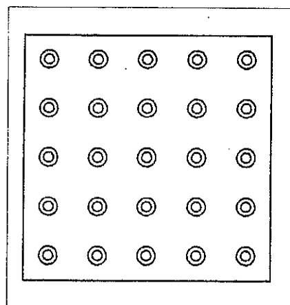
点字ブロックJIS点 300mm × 300mm
