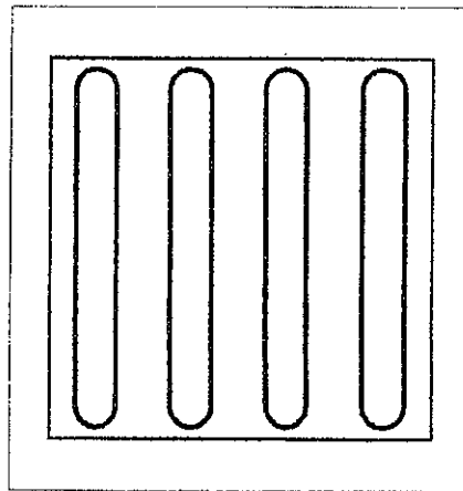
点字ブロック建設棒 300mm × 300mm
